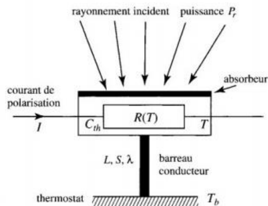
Figure 1 - Schéma d'un bolomètre
